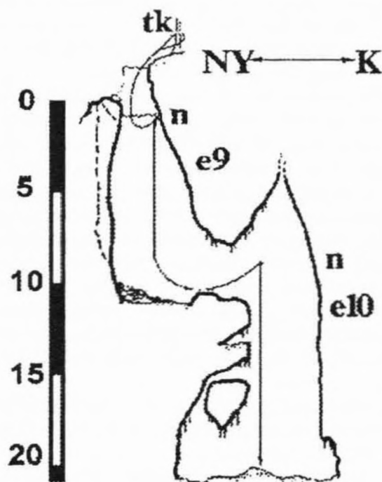
Komjádi Jég I.-zsombol (vázlatos hosszelvény)
