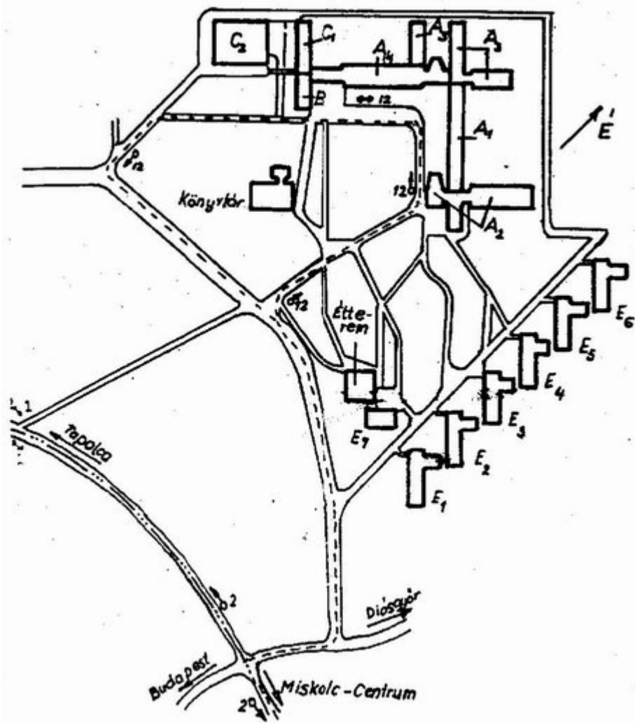
A NEHÉZIPARI MŰSZAKI EGYETEM ÁTTEKINTŐ ALAPRAJZA
