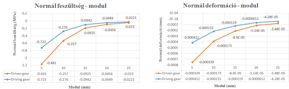
14. ábra. Kutatás: a modul változásának hatása a TCA paraméterekre [4]
