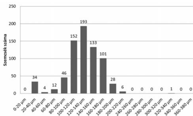
4. ábra: Az optikai mikroszkóppal mért darabszám szerinti szemcseméret-eloszlás adatai a kvarchomok 106-160 \mu\text{m} közötti frakció esetén
