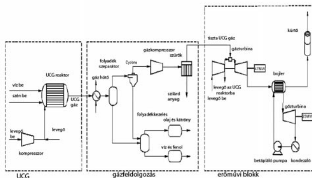
4. ábra: A Chinchilla Projekt elvi vázlatja [2]
