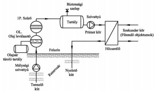
4. ábra: A példa rendszer elvi vázlatja
