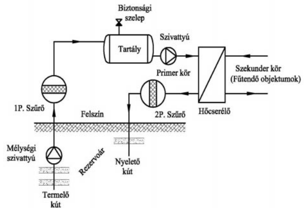
1. ábra: A földhő alapú távhőszolgáltatás elvi vázlata
