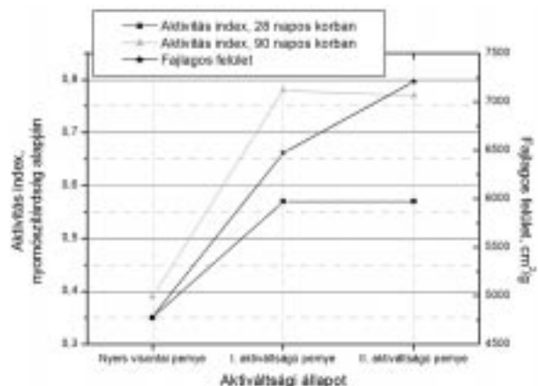
4. ábra: Aktivált és nem aktivált visontai pernyekötőanyag aktivitás indexe (nyomószilárdság alapján számított) és fajlagos felülete
