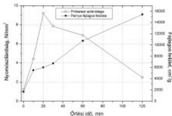
8. ábra: A pernye fajlagos felületének és a geopolimer szilárdságának változása az órlesi idő függvényében
