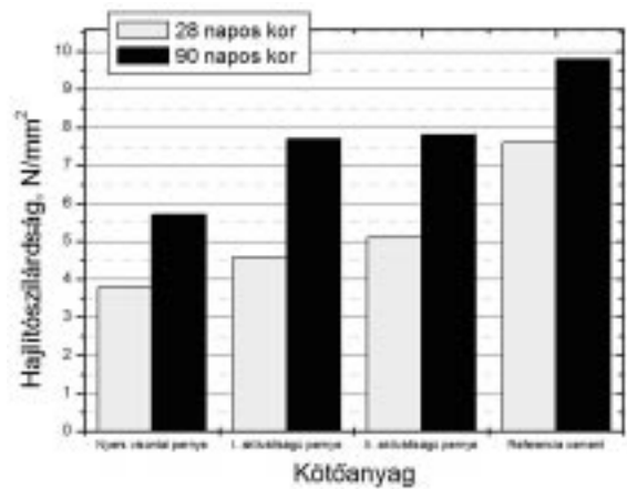
3. ábra: Habarcszásabok hajlítoszilárdságának változása az aktiváltsági állapot és a vizsgálati kor függvényében
