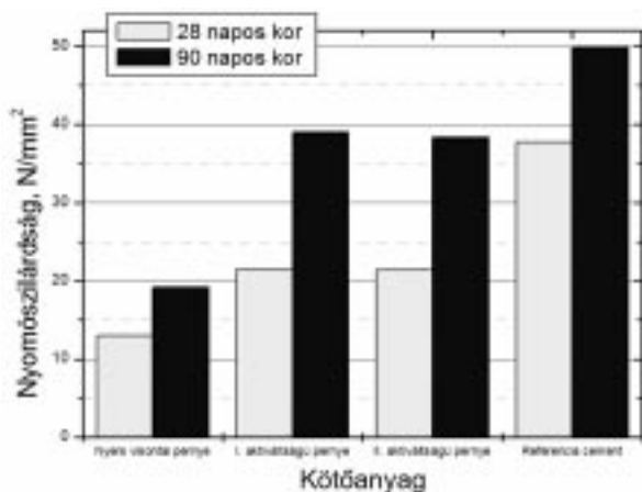
2. ábra: Habarcszásabok nyomószilárdságának változása az aktiváltsági állapot és a vizsgálati kor függvényében
