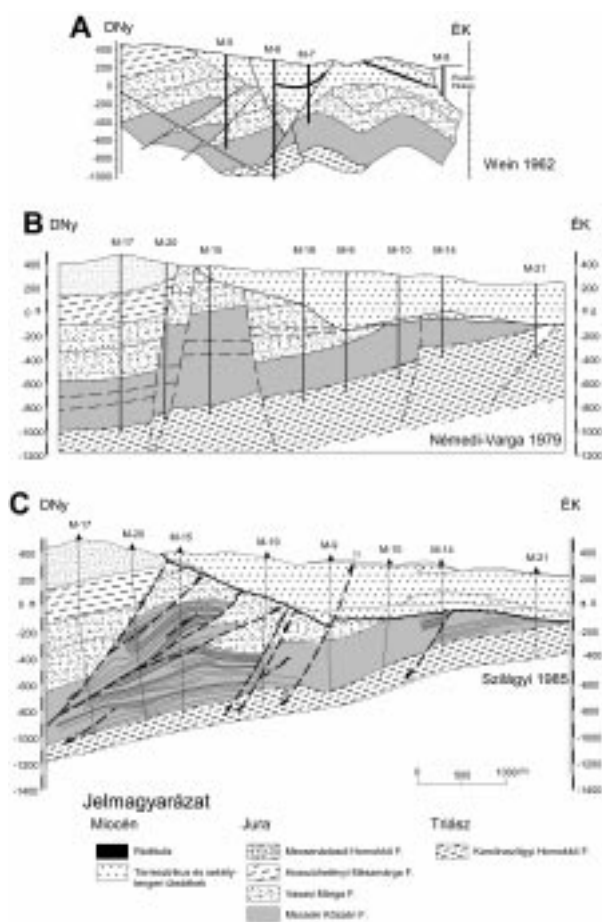
2. ábra: Maza-Dél dőlésirány szerinti földtani szelvénye Wein Gy. (1962), Némedi-Varga Z. (1979) és Szilágyi T. (1985) szerint
