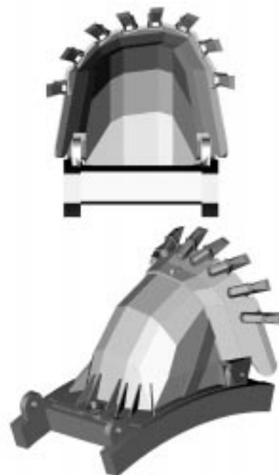
8. ábra: A VABE 1300-as géphez tervezett meríték
