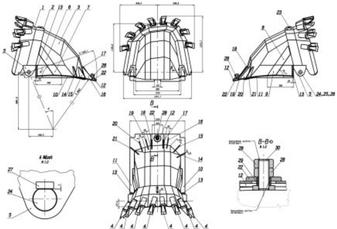
9. ábra: Zárt meríték összeállítási rajza
