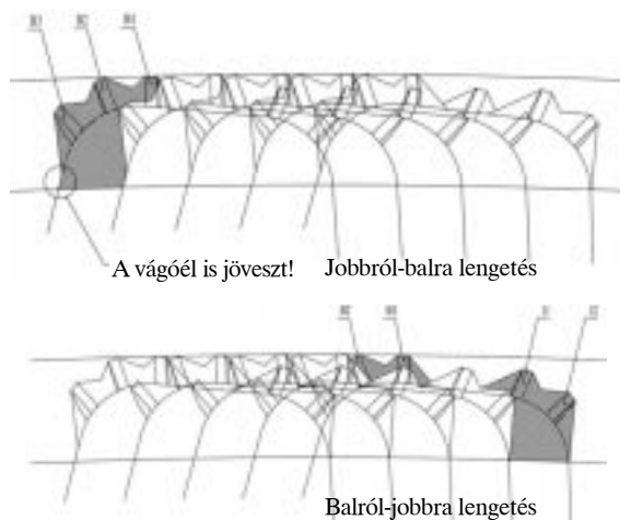
5. ábra: Forgácsképek az íves merítéknél, jól látszik az aszimmetrikus forgácskép ( t_{cmax}=0.6\text{ m} )
