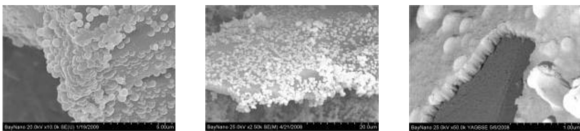
7. ábra: Szilícium-karbid szemcsék kémiai nikkellezése a) savas előkezelés, szárítás, kémiai nikkellezés b) felületi oxidáció, kémiai nikkellezés c) ón-kloridos érzékenyítés, palládium-kloridos aktiválás, szárítás, kémiai nikkellezés
