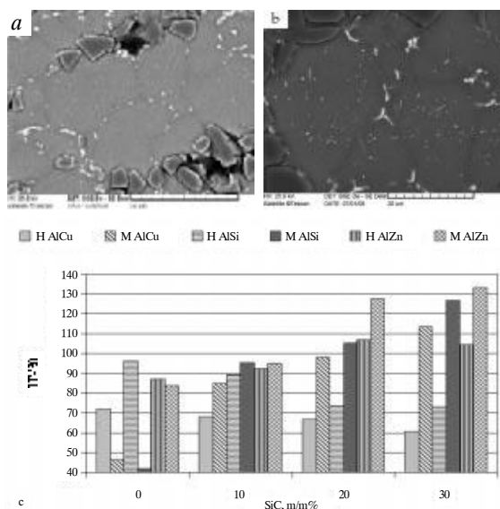
4. ábra: a) Hidegsajtó b) melegsajtó AlCu-30SiC kompozit SEM felvétele c) A kompozitok keménysége a SiC-tartalom függvényében (A SEM felvételeket Kovács Árpád készítette)
