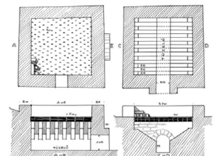
A III. JELZÉSŰ TÉGLÁÉGETŐ KEMENCE TÜZELŐ ÉS ÉLETŐNYELISÉGENEK ALAPRAIZAI A HOZZÁTARTÓZÓ HOSSZ-ÉS KERESZTMETSZETEKSEL
