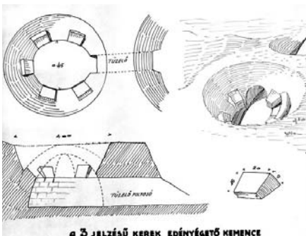
A 3. JELZÉSŰ KERESZTMETSZETŰ KEMENCE
