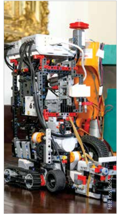
A robot vezetéséhez két pilótára, egy irányítóra és egy kábeltartó segítőre volt szükség
