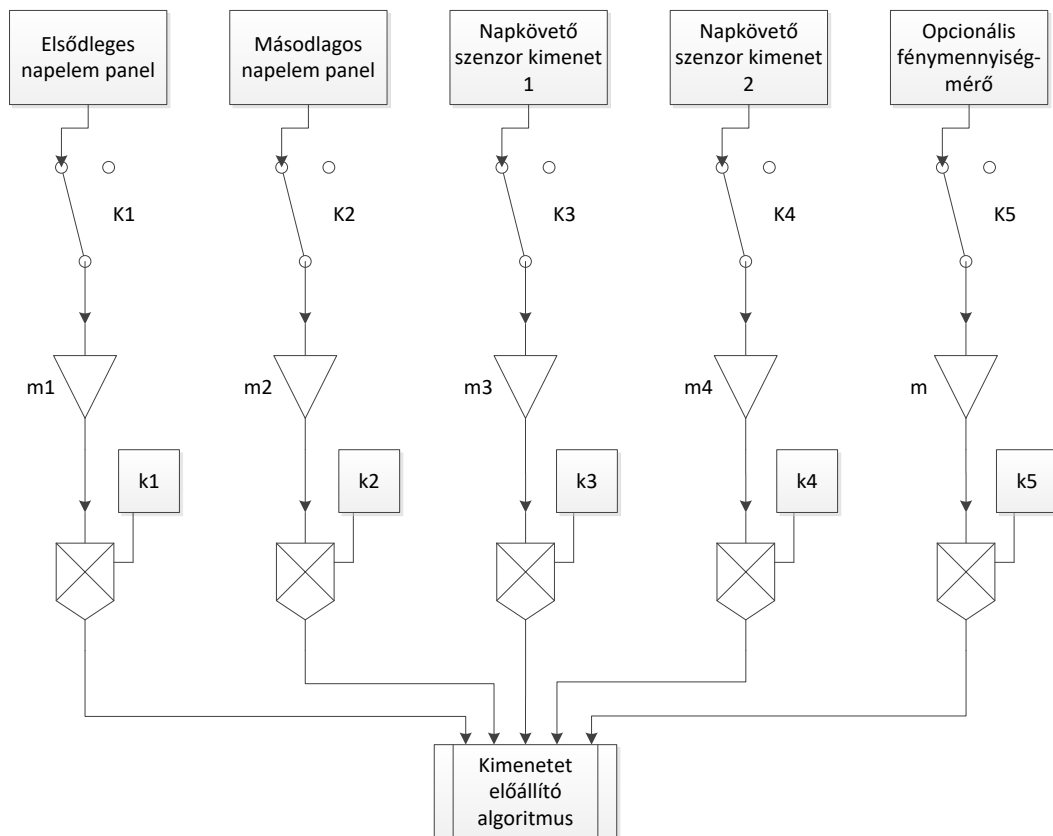
6. Ábra: Szoftveres fényerősség mérő algoritmus működési vázlat
