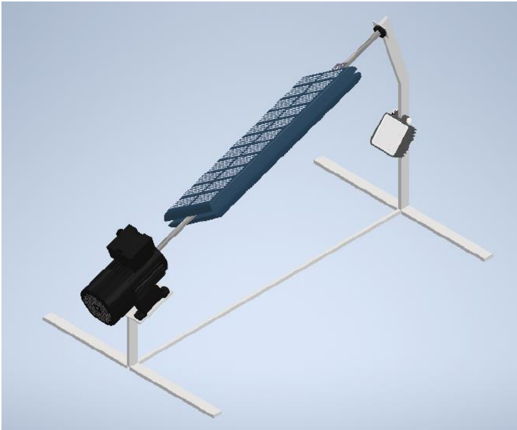
7. Ábra: Egytengelyes forgási mechanizmussal rendelkező redundáns napelem panel izometrikus ábrája
