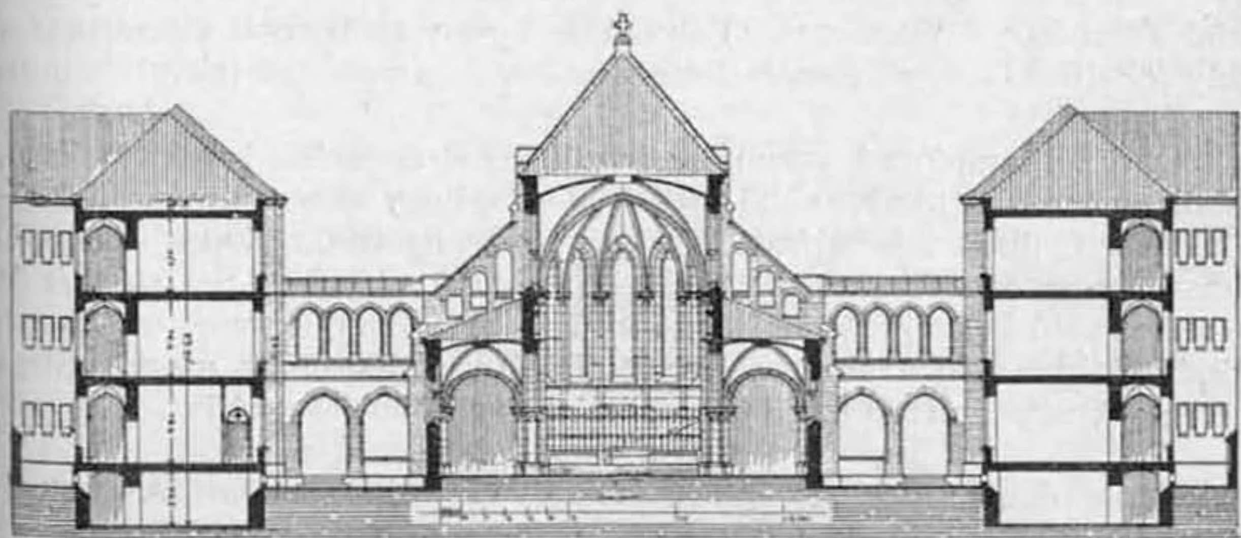
Aigner Sándor pályaművének keresztmetszetei.
