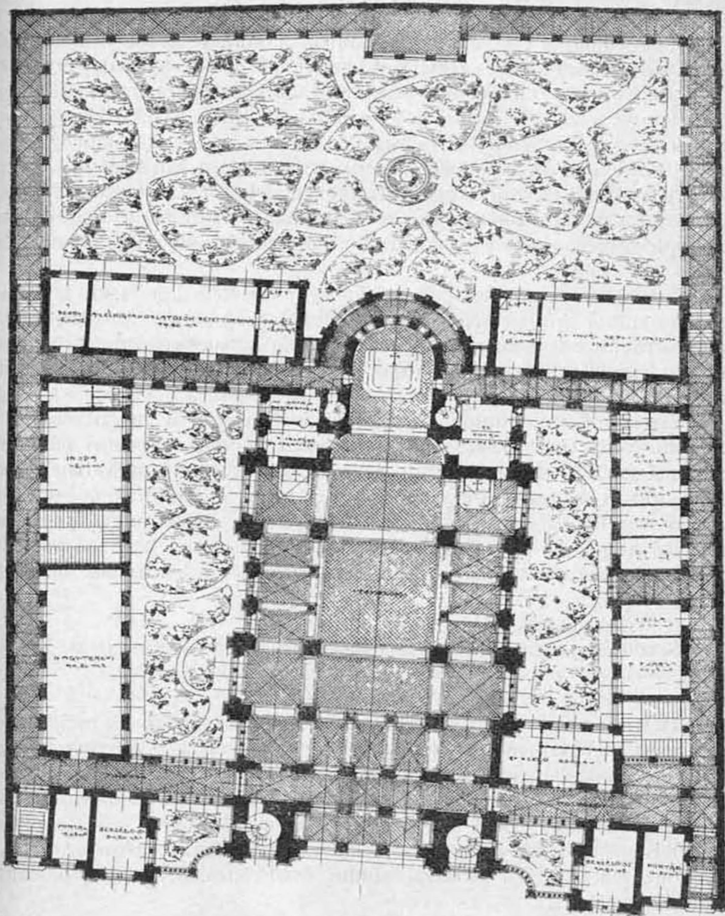
Hofhauser Antal pályaművének alaprajza.
