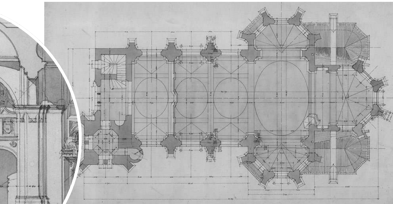
A felsőrönöki Szent Imre-templom tervrajzai, 1898.
