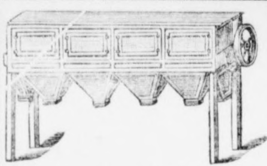
Lisztosztályozó henger.
