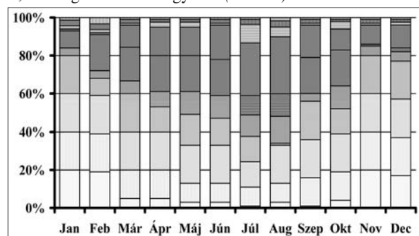
3. ábra Az ALADIN modell esetében használt 10 különböző réteg relatív nedvességének globál sugárzást csökkentő hatása (09 - 15 UTC) Pontozott: Alacsony szintű Függőleges csíkozás: Középmagas szintű Függőleges csíkozás: Magassintű felhőzet (lásd a szövegben)
