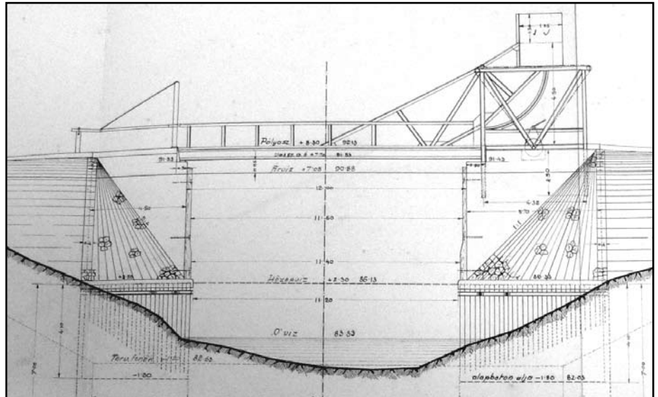
A Jösch tervezte híd a jobb (szigeti) oldalon fogazott ível kapcsolódott, nyitott helyzetben állása teljesen függőleges
