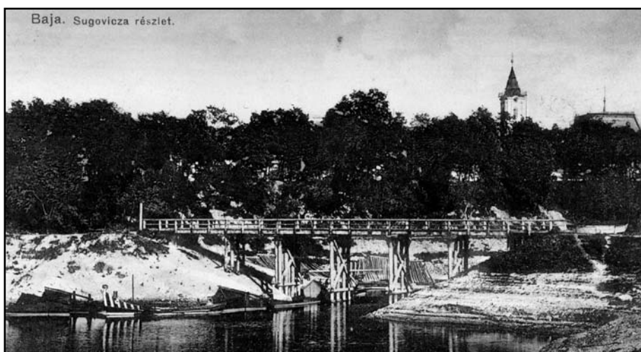
A hatnyílású fix-híd vagy járomhíd 3,6 méter széles volt
