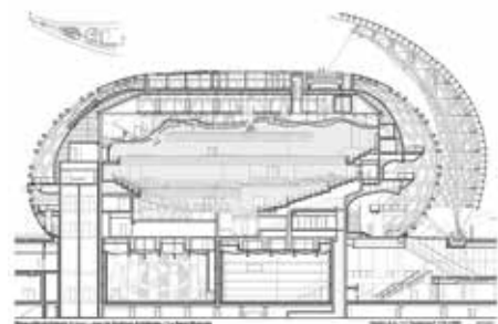
► Hosszmetszet az auditóriumon keresztül
