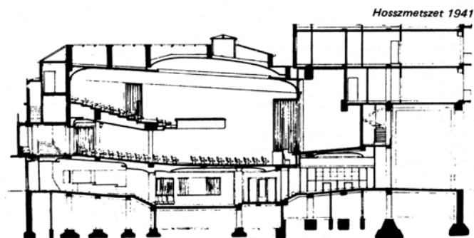
Hosszmetszet 1941
