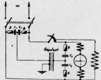
Egyenáramú mellékáramkörű motor zavarszűrése.
