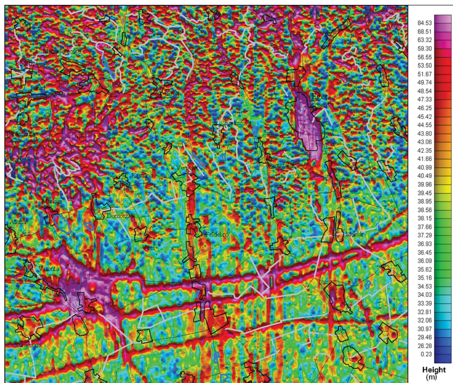
12. ábra | Az egri mérési terület (K-Mátra és Ny-Bükk) repülésmagasság-térképe Figure 12 | Flight height map of Eger exploration area
