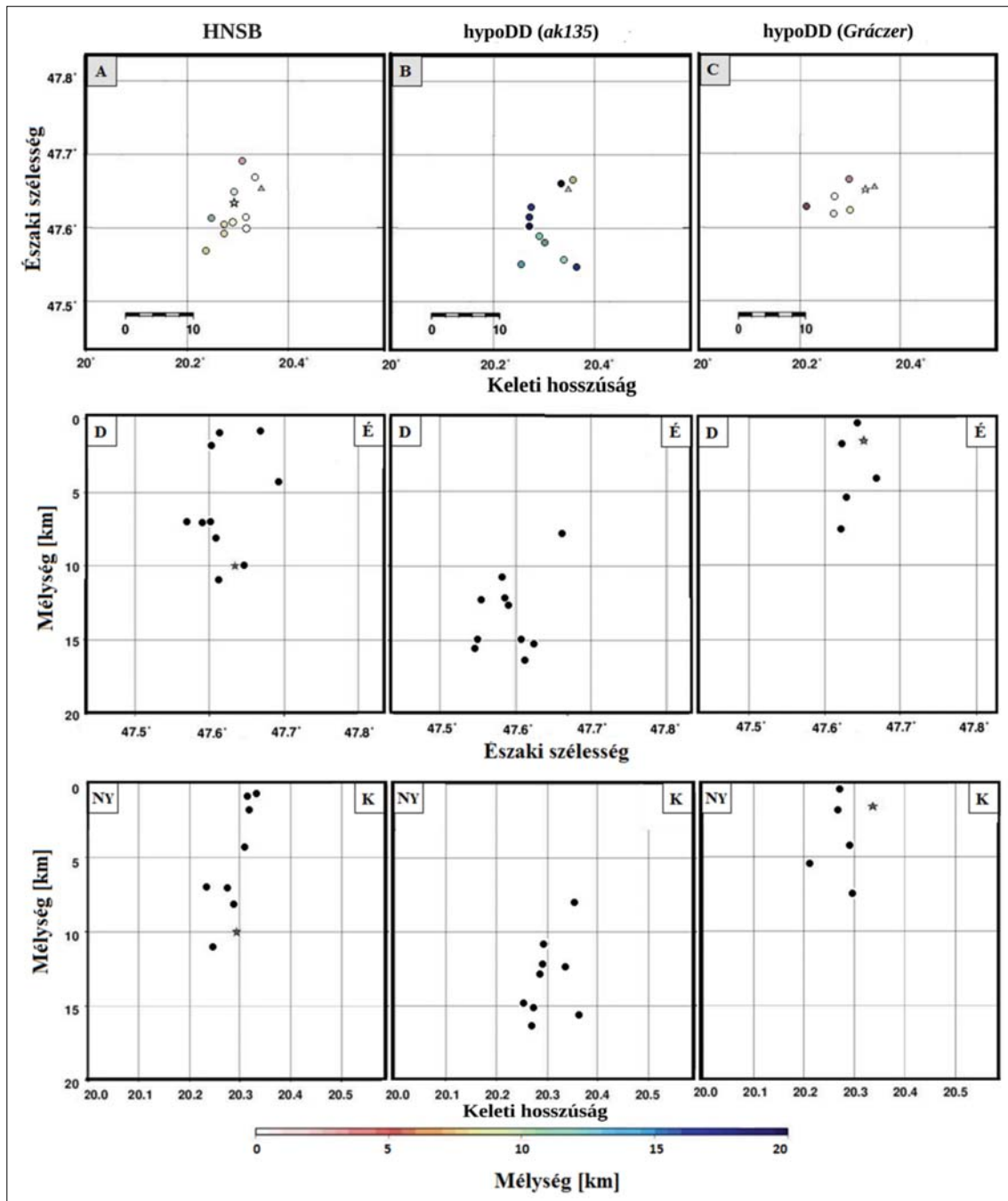
4. ábra Hipocentrumok térképi nézetű (felső sor), D–É mélységshelvényei (középső sor), NY–K mélységshelvényei (alsó sor). A) Kövesligethy Radó Szeizmológiai Obszervatóriumban rutinszerűen meghatározott hipocentrumok, B) az ak135 1D-s sebességmodellel számított abszolút hipocentrumok hypoDD-megoldásai, C) a Grácz-féle 1D-s sebességmodellel számított abszolút hipocentrumok hypoDD-megoldásai. A szín-skála a fészekmélységeket, a csillag a főrengést jelöli
