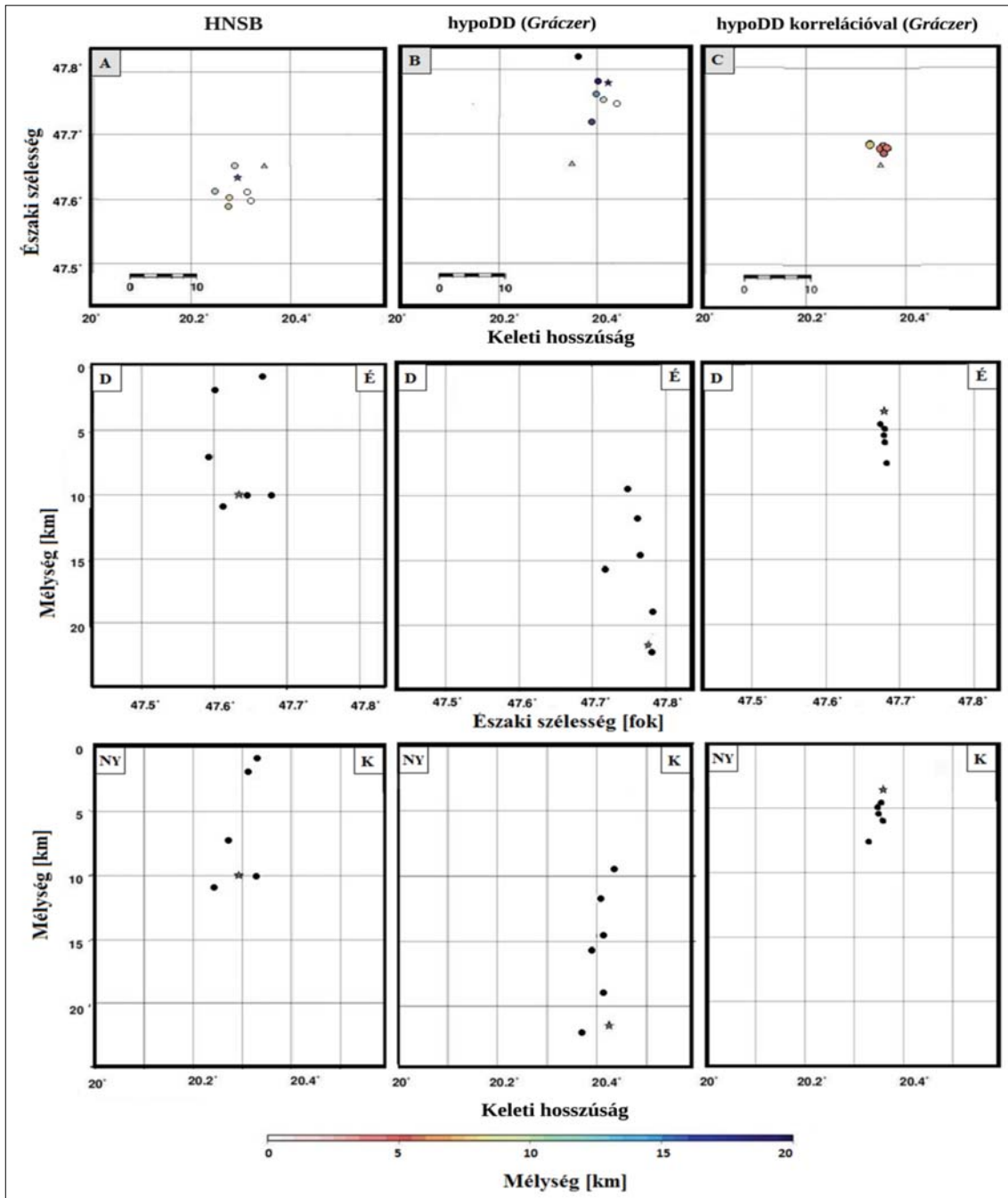
8. ábra Hipocentrumok térképi nézetei (felső sor), D–É mélységszelvei (középső sor), NY–K mélységszelvei (alsó sor) ismételt fáziskimérések, valamint hullámforma-korreláció után. A) Kövesligethy Radó Szeizmológiai Observatóriumban rutinszerűen meghatározott hipocentrumok, B) a Gráczter-féle 1D-s sebességmodellel számított abszolút hipocentrumok hypoDD-megoldásai, C) a Gráczter-féle 1D-s sebességmodellel számított abszolút hipocentrumok hypoDD-megoldásai a differenciális időekkel. A színskála a fészekmélységeket, a csillag a főrengést jelöli
