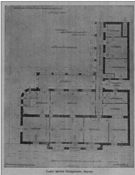
A Kállay-ház alaprajza (Építészeti Szemle)
