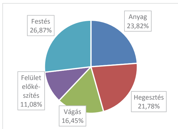
7. ábra. Költség eloszlás k_f/k_m=2 esetén, lézer hegesztés, lézer vágás esetén
