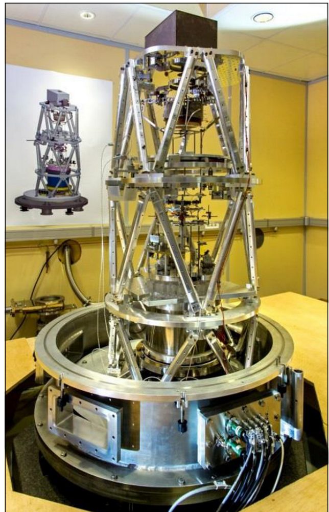
15. ábra. A kilogramm-alapegység számára összehasonlító (referencia) mérésként szolgáló, ún. Kibble-mérleg látképe
