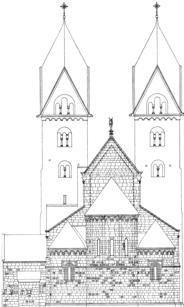
Kőfalvi Imre felmérési rajza a keleti homlokzatról.
