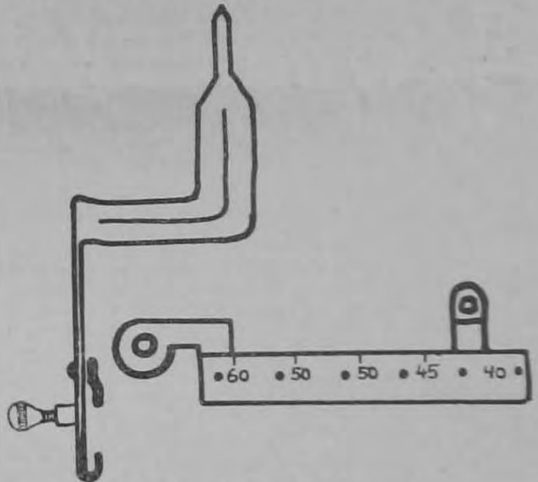
35. ábra: A célzótűske és az irányzósín.
