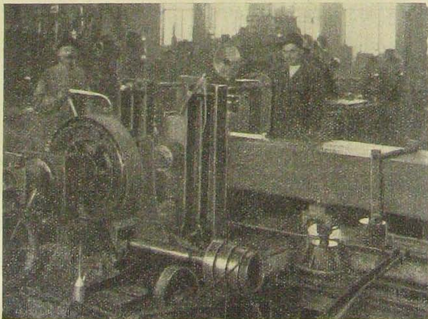
A láncztagok együttes furása.
