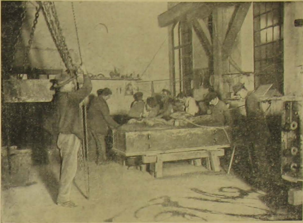
Az eredeti gipszmintát kiformázzák homokban.
