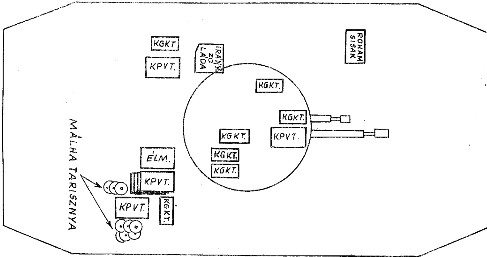
A PSZH belső málházásának elvi vázlata
