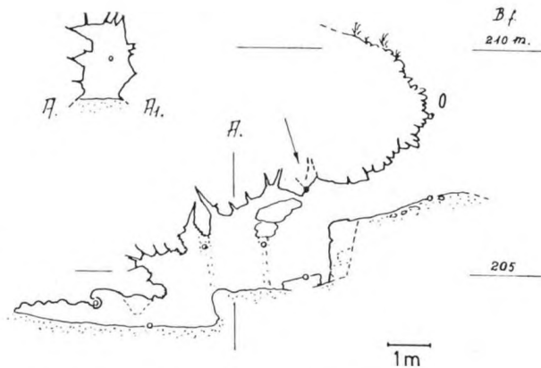
A Zsindely utcai-barlang hosszszelvénye Készítette: Horváth J. és ifj. Cseh S.
