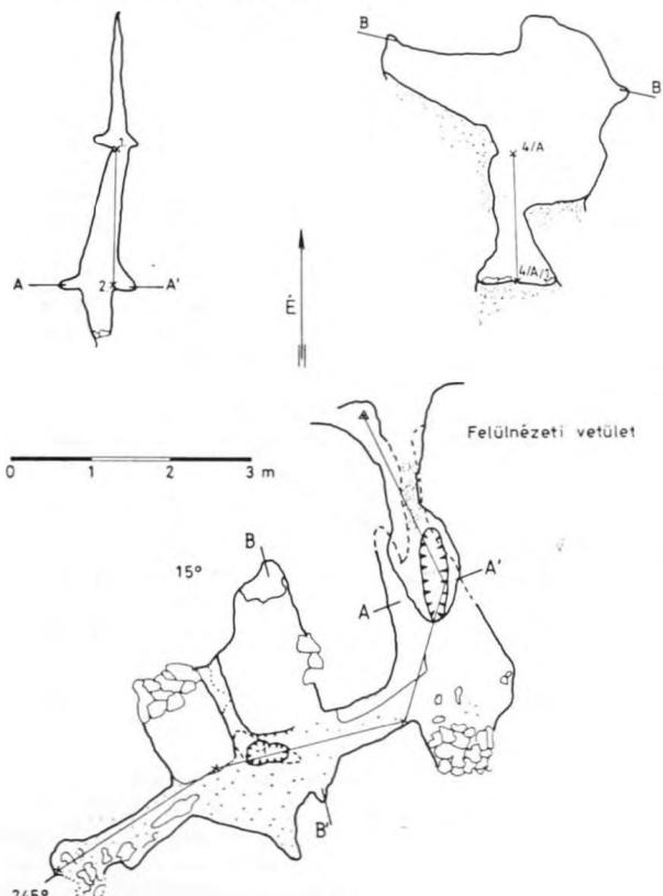
A Franciabánya 4. sz. barlangja (Felmerte: Rose Gy.)
