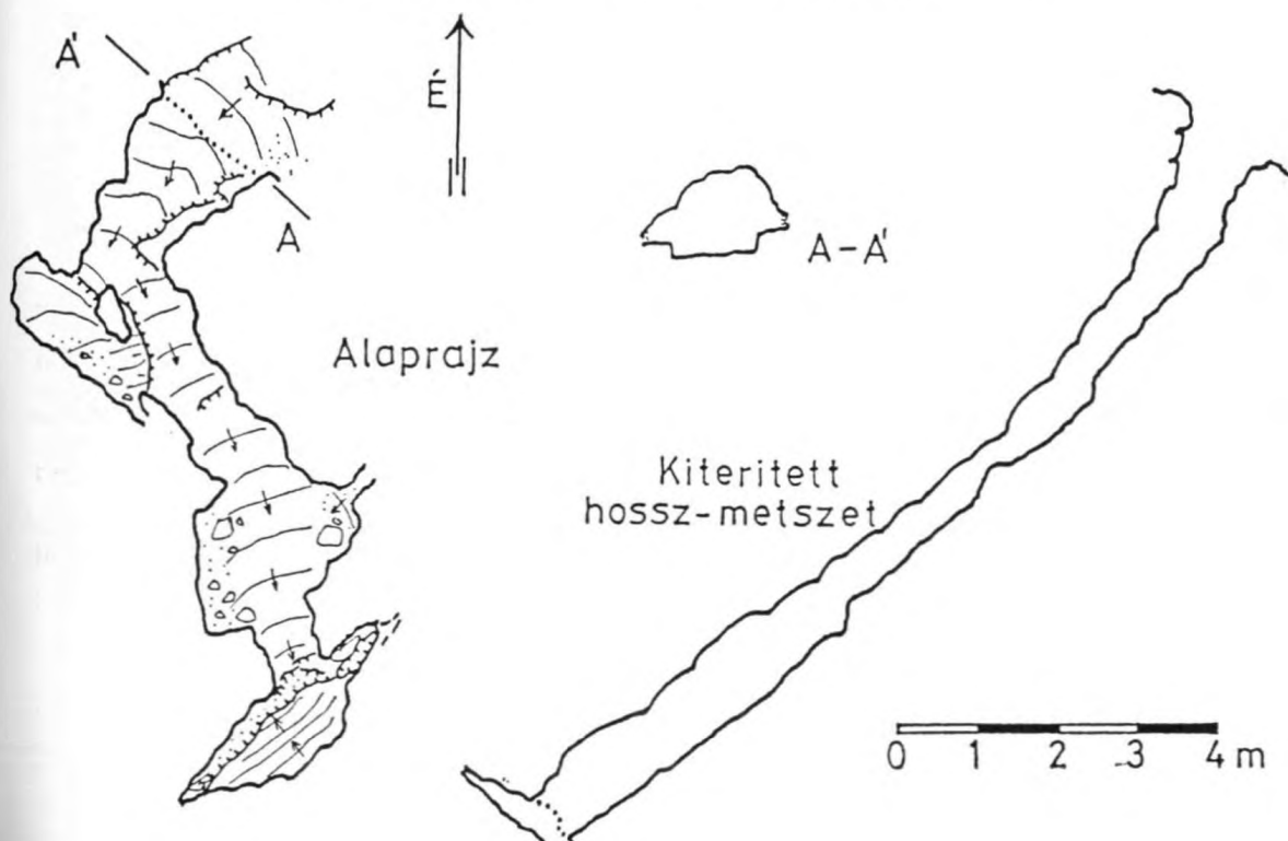
A Korallos-barlang . Készítette: Juhász M. (Barlangtani Intézet)
