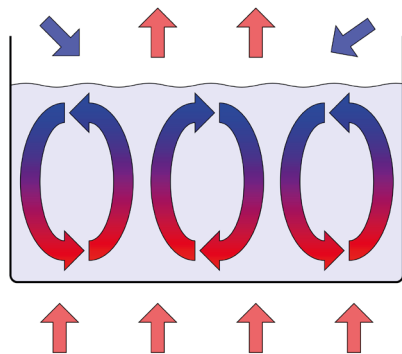
7. ábra. Alulról melegített, felülől hűtött folyadékban kialakuló, cellás szerkezetű áramlás képe. A folyadék hőmérsékletét és áramlásának irányát megfelelő színű nyilak jelzik (a piros szín a melegnek, a kék a hidegnek felel meg). Az edény alatti és feletti nyilak a melegítést és hűtést jelképezik
