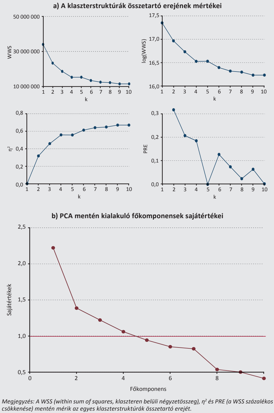
6. ábra A PCA és a k-közép klaszterelemzés ábrái
