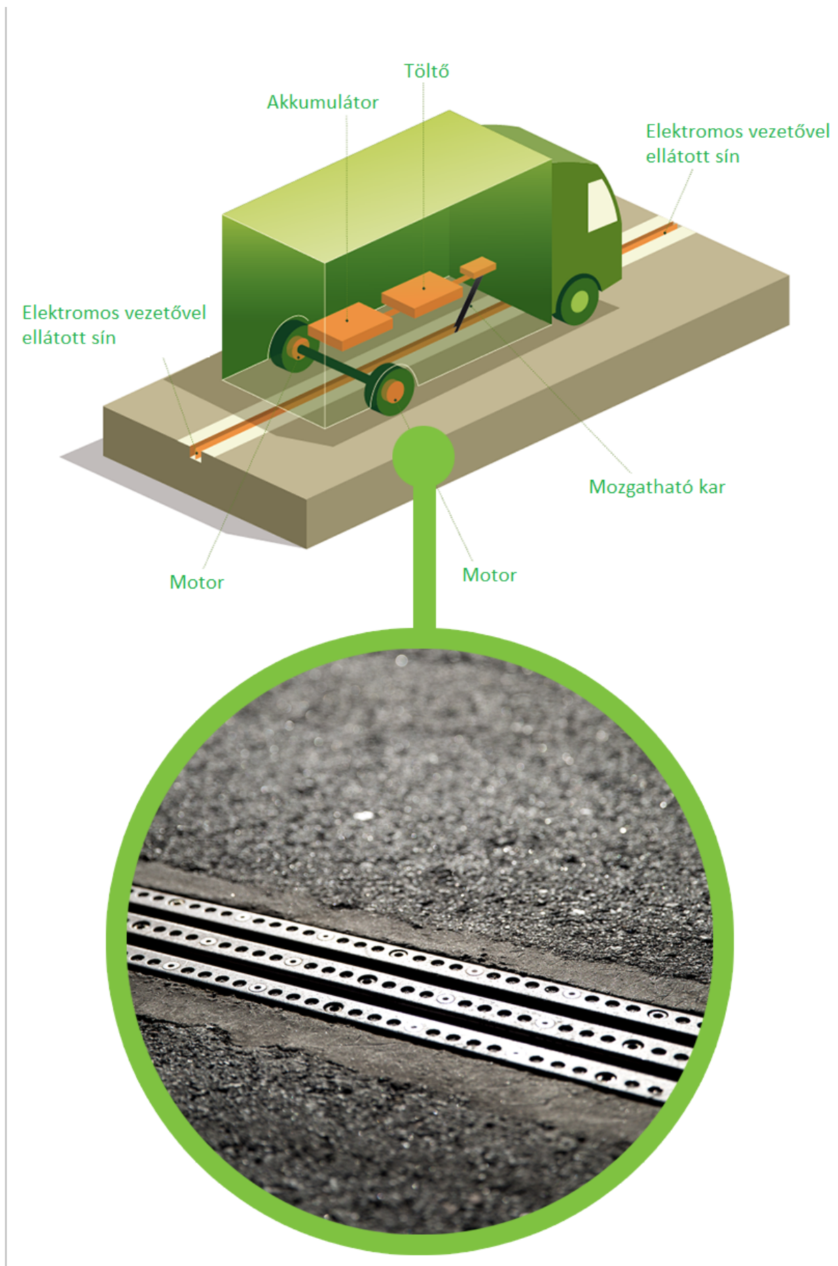
2. ábra eRoad Arlanda projekt műszaki megoldása
