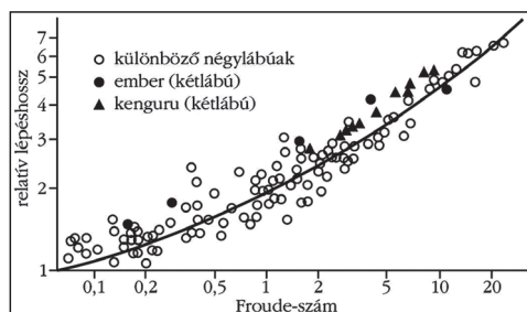
4. ábra. Az r = s/L relatív lépéshossz az f = u^2/(gL) Froude-szám függvényében, ahol g a földi nehézségi gyorsulás, u az állat mozgássebessége, L a láb hossza, s pedig a lépéshossza 3
