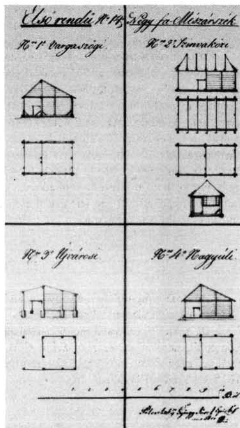
22. kép. Az uradalmi kezelésű négy mézárszék (Varga-szögi, Szinva-közi, Újvárosi és Nagyúti) alaprajza, ill. metszete
