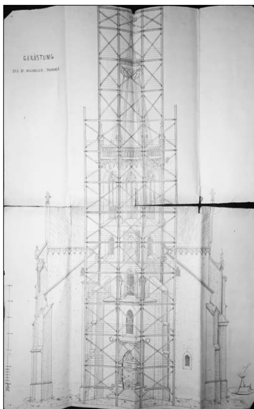
18. kép. A torony beállványozásának terve. Franz Mechle, 1865 (MNL GyMSMSL, IV. 1106. Fasc. XXV. No. 13957.)
