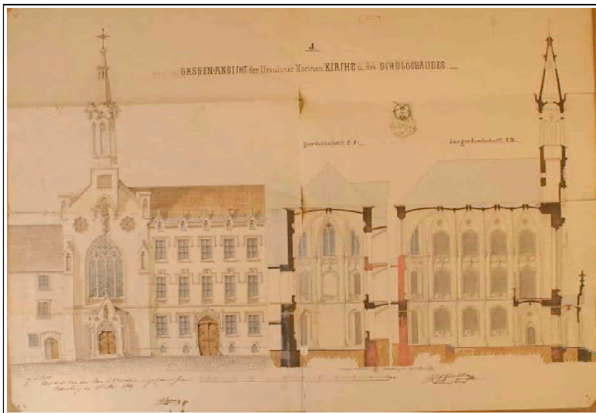
1. kép A templom és az iskola terve 1859-ből (Soproni Levéltár Fasc. XXIV. 5555/1862)
