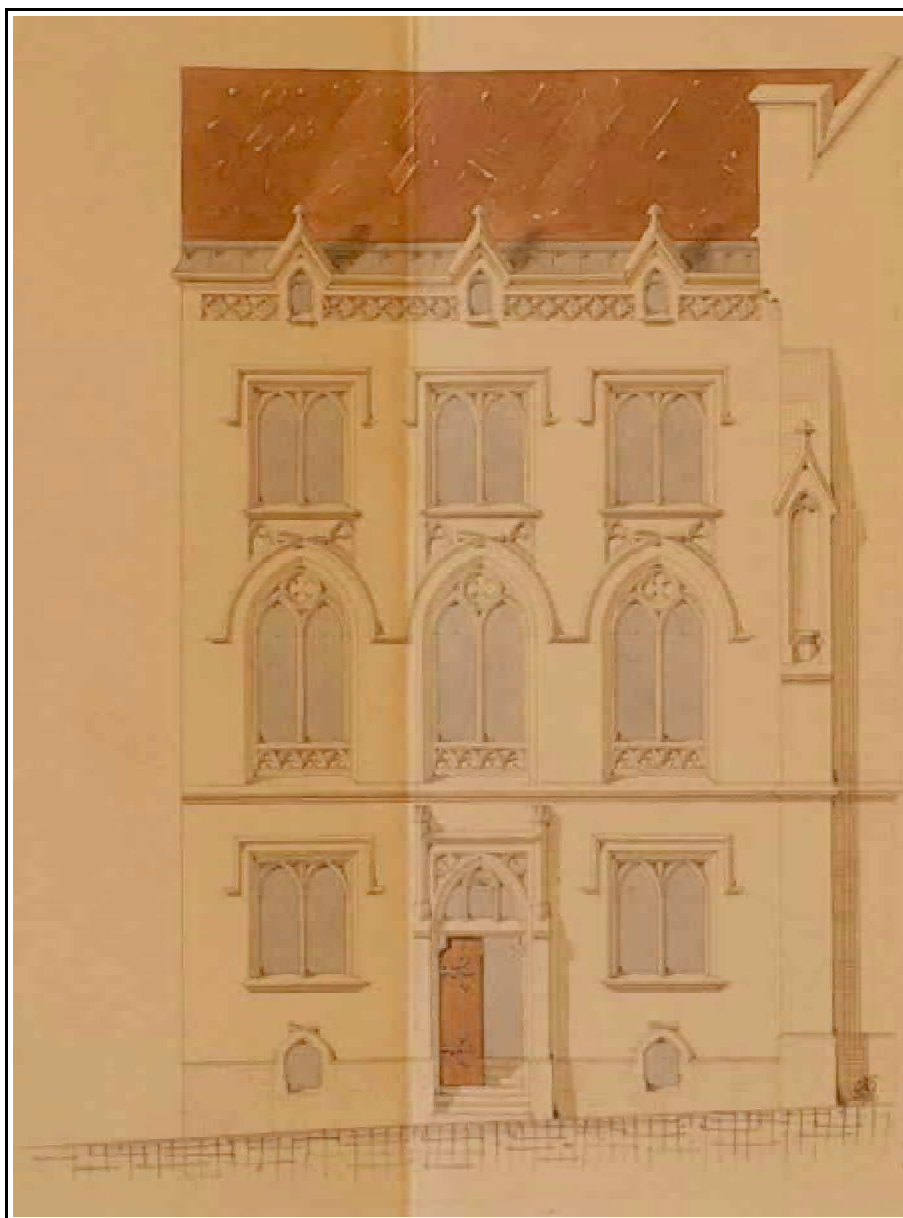
2. kép A zárda terve 1862-ből (Soproni Levéltár Fasc. XXIV. 5555/1862)
