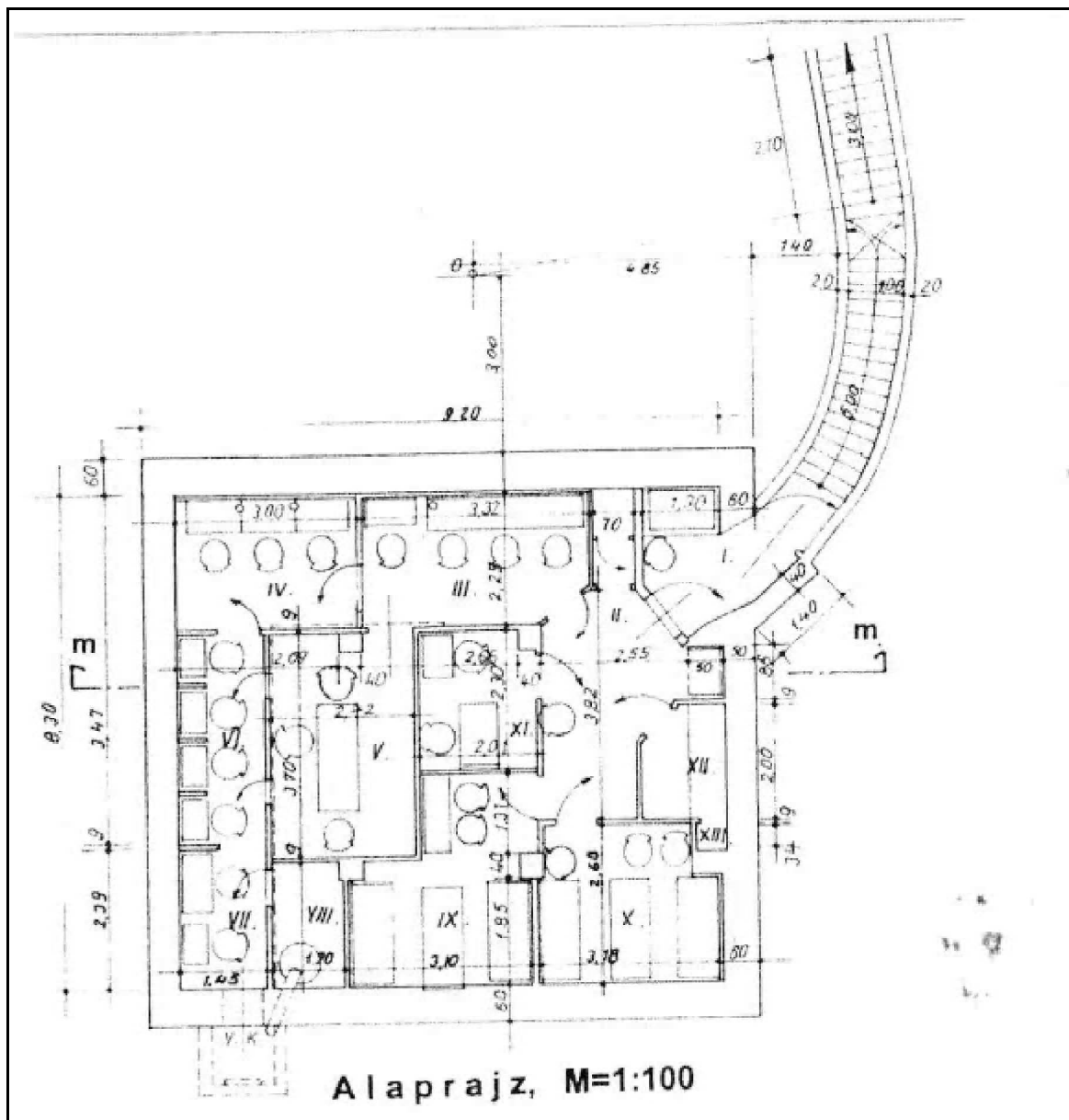
1. kép. A soproni Légoltalmi Parancsnokság óvőhelyének alaprajza
