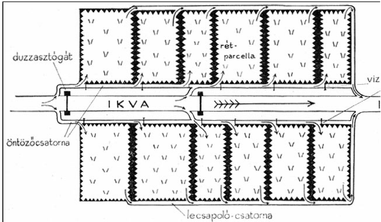
Az öntözési rendszer vázlat. Lovas Gyula rajza
