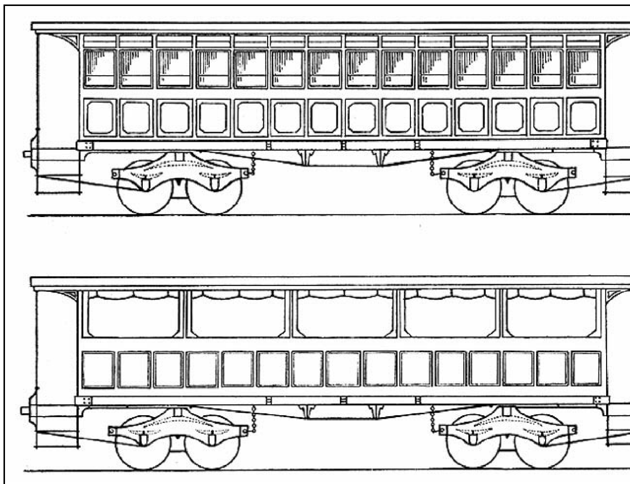
A Sopron–Bécsújhely-i vasút forgalmát lebonyolító gloggnitzi társaság négytengelyes személykocsijának jellegrajza
