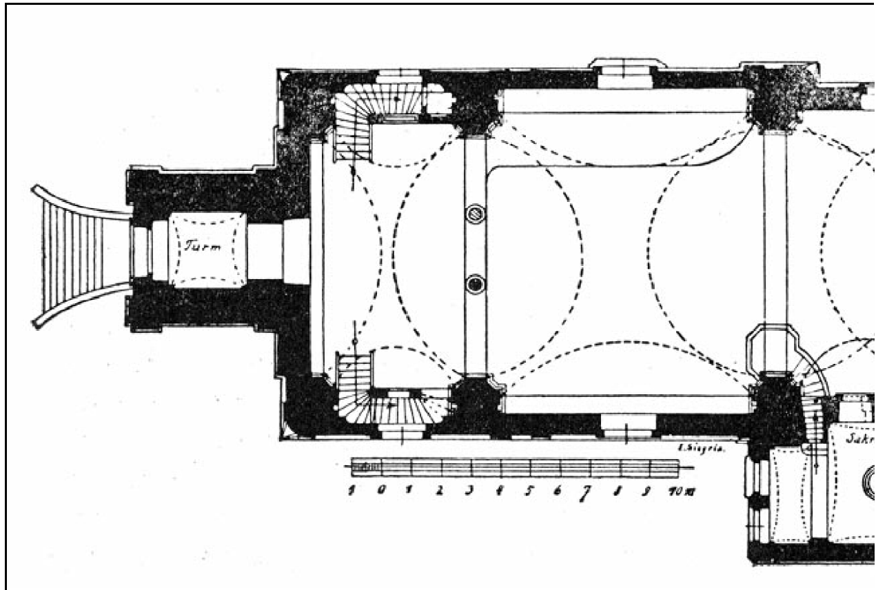
A ruszti evangélikus templom alaprajza. (Neumayer Lőrinc tervezése.)
