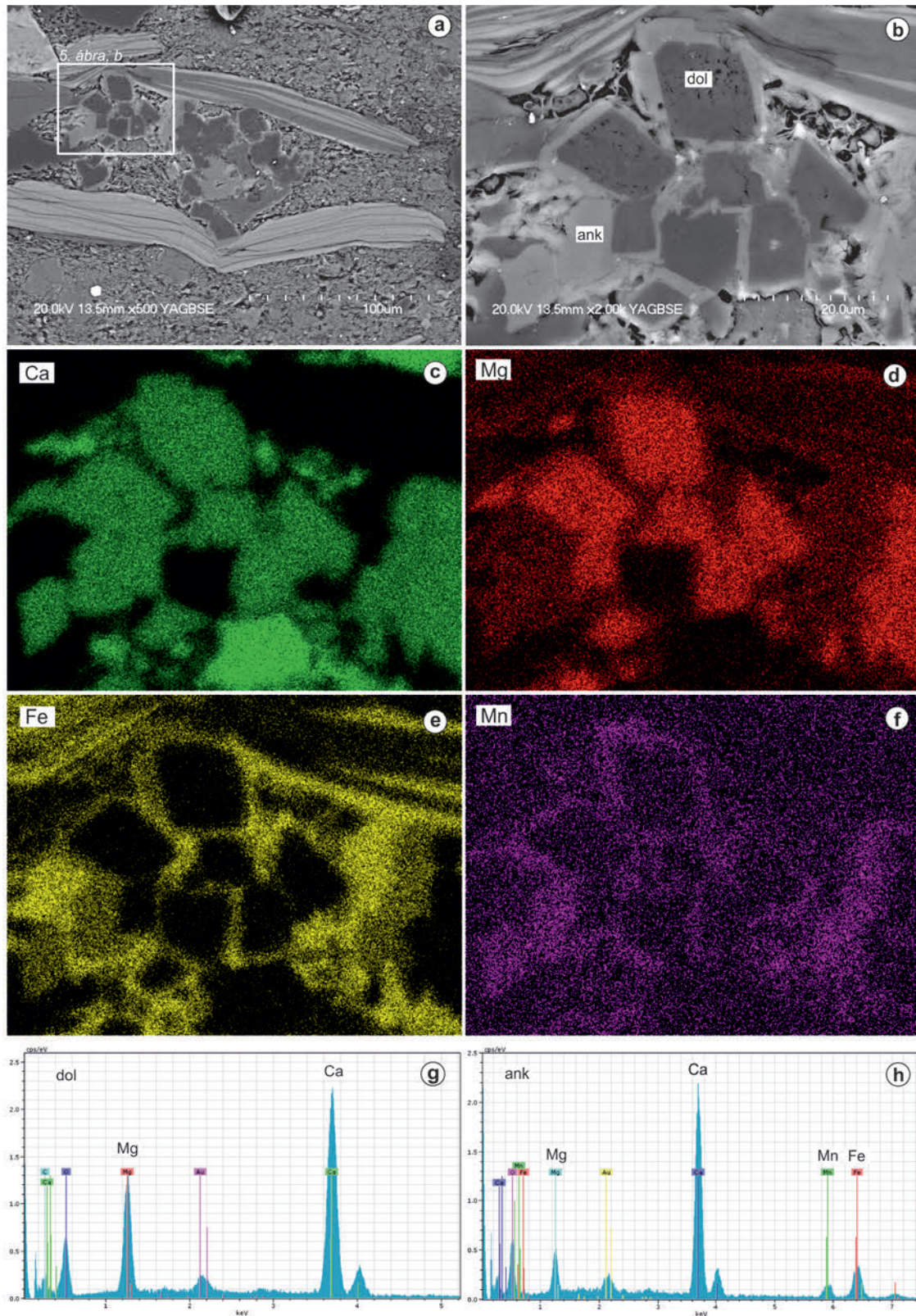
5. ábra. A 35/10 minta (Hódmezővásárhely-I fúrás, 5167,0–5183,0 m) karbonátfázisának kémiai összetéti jellemzői elektronmikroszkópi vizsgálatok alapján. a) Romboéderees kristályokból álló dolomithalmazok Fe-dolomit/ankerit továbbnövekedéssel (visszaszórt elektronkép, SEM/BSE); b–f) Dolomitkristályok (dol) körüli ankerit (ank) továbbnövekedés (visszaszórt elektronkép, SEM/BSE, illetve SEM/EDS elem térképek); g) és h) A dolomitkristályok (dol) és ankerit (ank) továbbnövekedésük SEM/EDS energiádiszperzív spektruma (energia-beütésszám)
