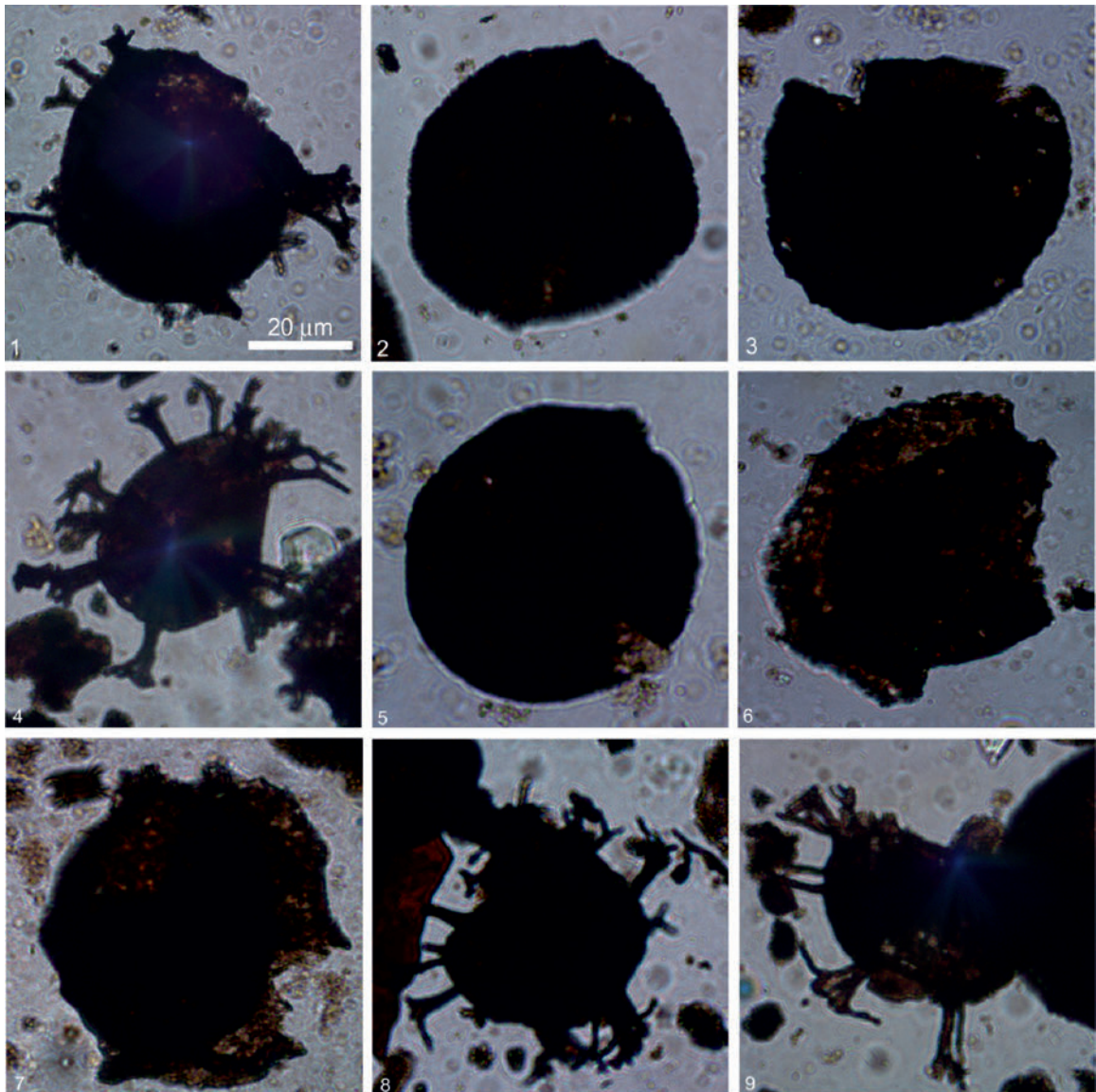
8. ábra. Jellemző dinociszták a Hódmezővásárhely–I fűrés vizsgált mintáiból (35. magfűrés). Az 1. képen szereplő méretarány 20 µm (mindegyik fotóra vonatkozik). 1. Spiniferites bentorii pannonicus SÜTÓNÉ SZENTAI 1986 (35/13); 2. Pontiadinium obesum SÜTÓNÉ SZENTAI 1982 (35/18); 3. Chytroeisphaeridia tuberosa SÜTÓNÉ SZENTAI 1982 (35/13); 4. Spiniferites bentorii oblongus SÜTÓNÉ SZENTAI 1986 (35/24); 5. Virgodinium asymmetricum SÜTÓNÉ SZENTAI 2010 (35/4); 6. Spiniferites balcanicus SÜTŐ-SZENTAI 2000 (35/4); 7. Spiniferites paradoxus (COOKSON & EISENACK, 1968) SARJEANT, 1970 (35/7); 8. Spiniferites bentorii coniunctus SÜTŐ-SZENTAI 1990 (35/4); 9. Spiniferites maisensis SÜTŐ-SZENTAI 1994 (35/4)
