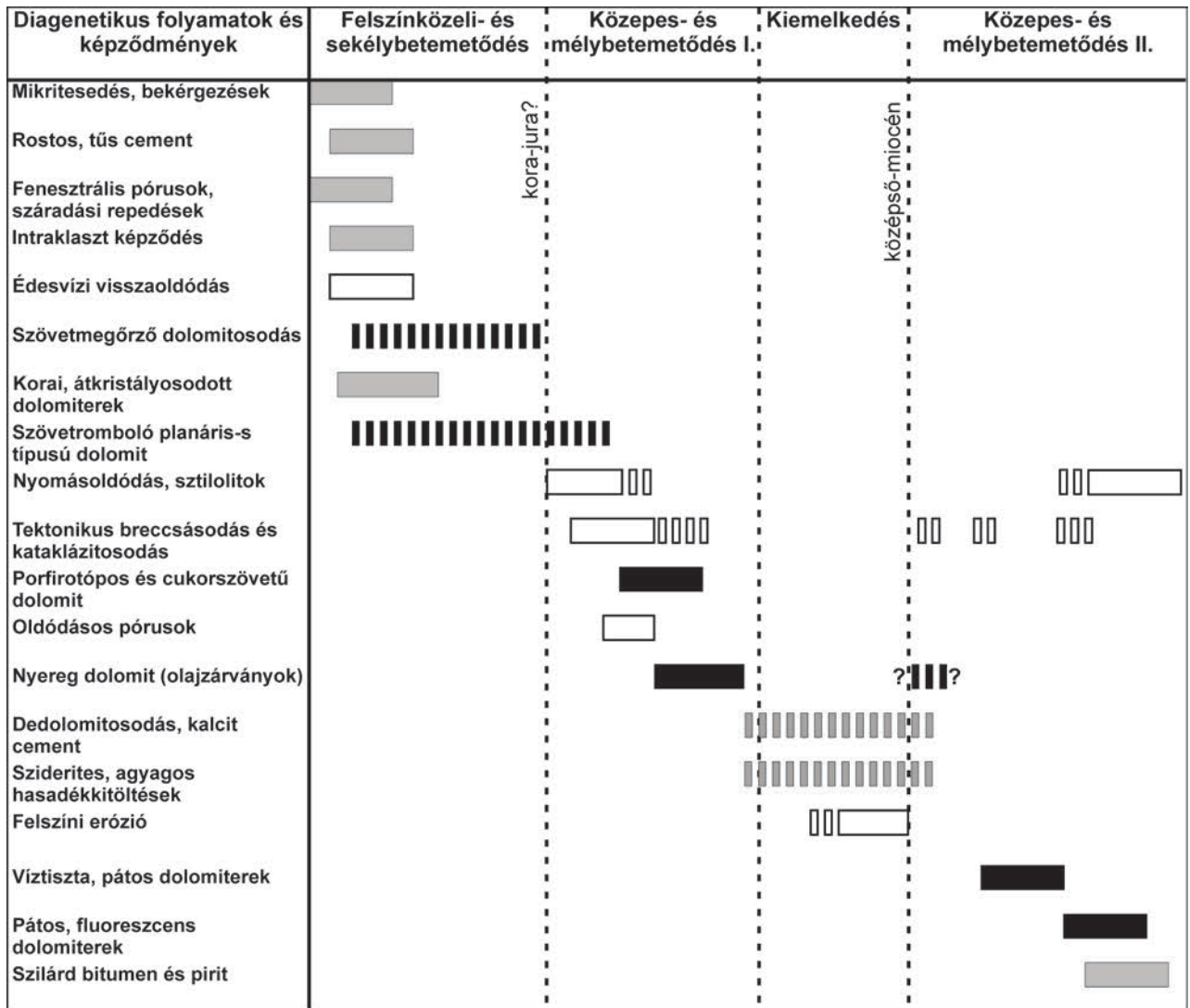
8. ábra. A Szegei Dolomit Formáció képződményeinek paragenetikai sorrendje. A fekete téglalapok különféle dolomitokat jelölnek, az üres téglalapok jelölik a töréses és oldódásos eseményeket, a szürke négyszögek pedig az egyéb diagenetikus képződményeket vagy folyamatokat
