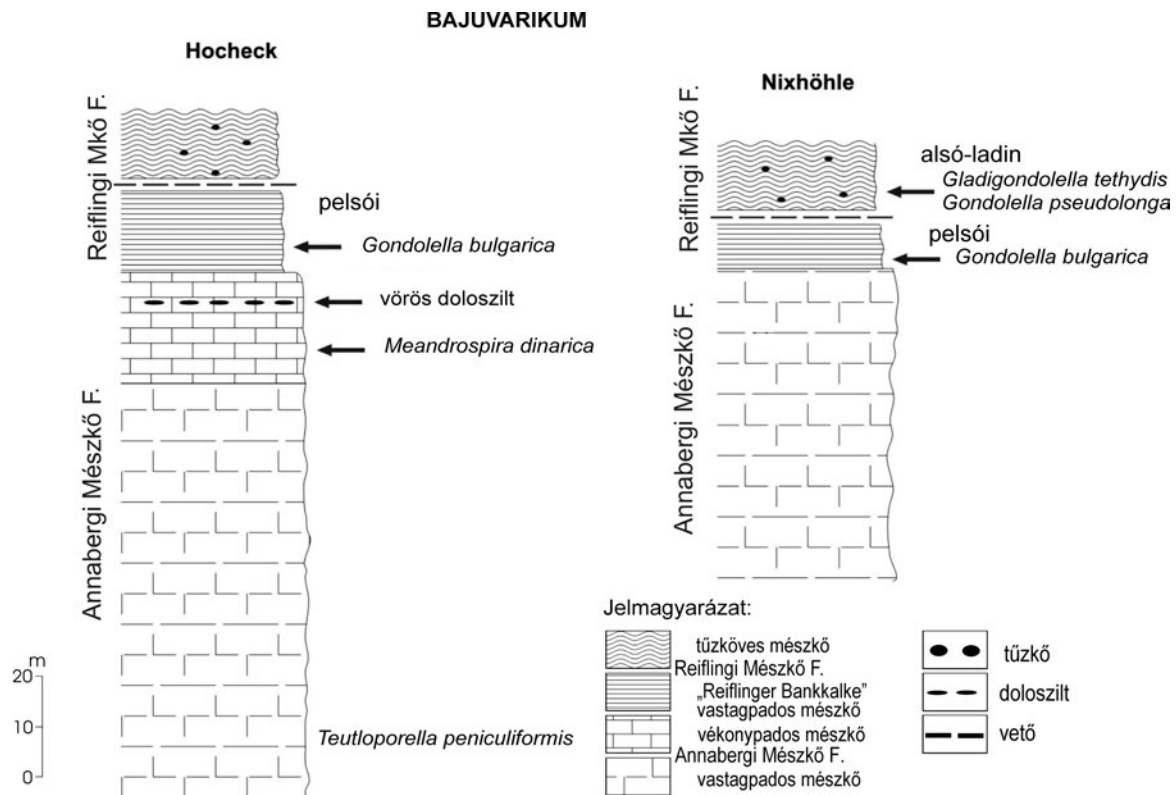
4. ábra. Vizsgált szelvények a Bajuvarikumból (Hocheck, Nixhöhle) Mintaszámok: Hocheck: Teutoporella peniculiformis A210, Meandrospira dinarica A208, Gondolella bulgarica A205 Nixhöhle: Gondolella bulgarica : A1063, G. pseudolonga , Gladigondolella tethydis : A1062
