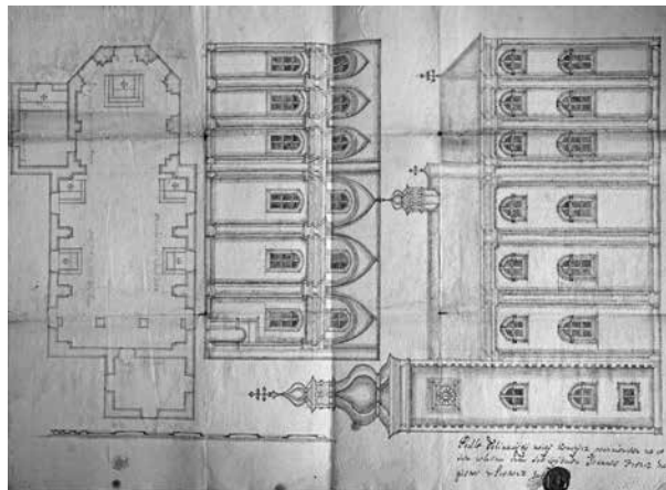
4. Johannes Francz eperjesi mester: A templom részben megvalósult átépítési terve, 1714, 1747 Arcibiskupský Archiv v Košiciach–Archivum Archidioecesis Cassoviensis. Košické biskupstvo. Parochialia. Acta Parochiae Tallya. Delineatio Ecclesiae Tallyensis, 1714, 1747
