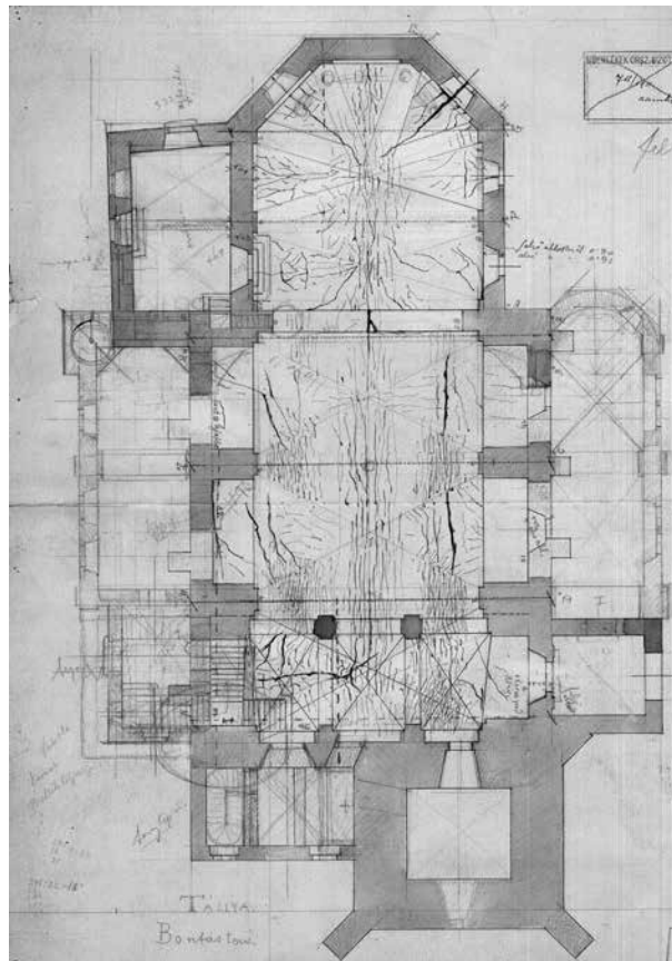
6. Stehlo Ottó: Bontási terv, 1911. Magyar Építészeti Múzeum és Műemlékvédelmi Dokumentációs Központ, Tervtár, ltsz. R 7758.
