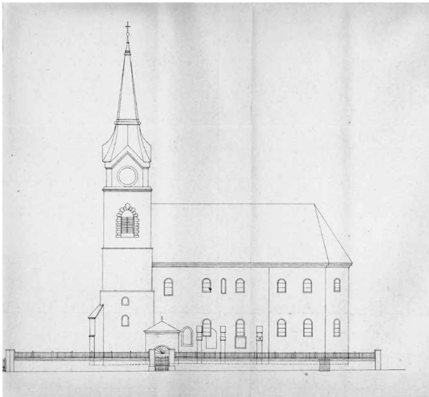
2. A templom déli homlokzata. BME építészmérnök hallgatók nyári városfelmérései, 1993 Magyar Építészeti Múzeum és Műemlékvédelmi Dokumentációs Központ, Tervtár, ltsz. D 36973
