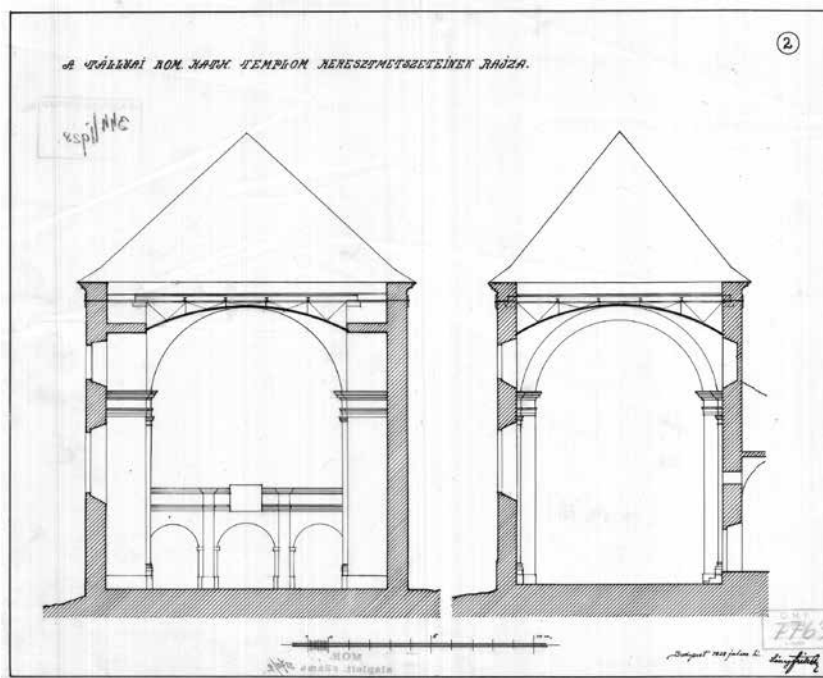
7. Lácza Fritz Oszkár: A hajó és a szentély keresztmetszete a tervezett rabicboltozattal, 1928 Magyar Építészeti Múzeum és Műemlékvédelmi Dokumentációs Központ, Tervtár, Itsz. R 7763.
