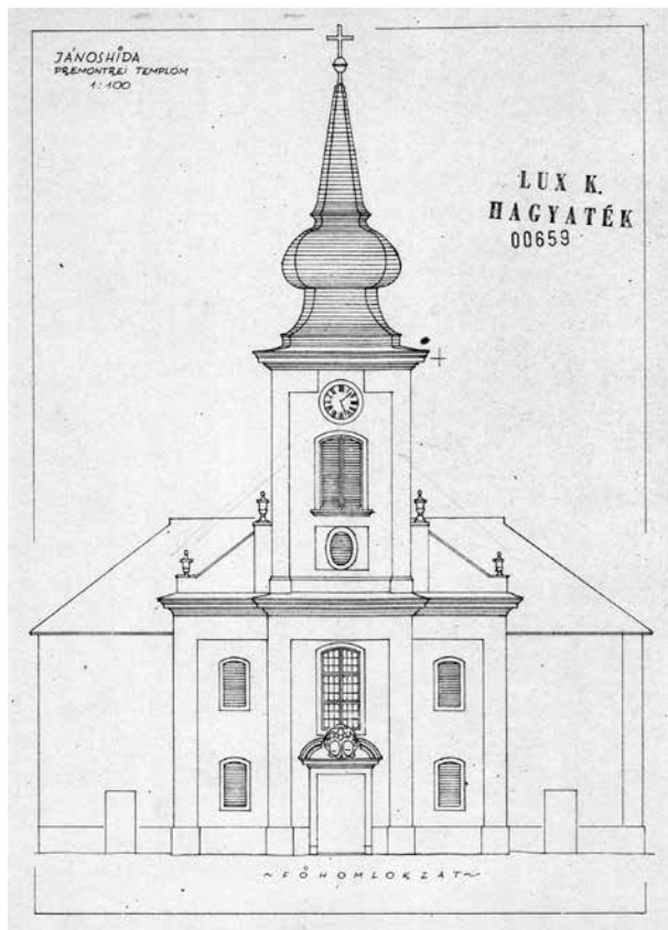
4. Lux Kálmán: A jánoshidai volt premontrei prépostsági templom bővítési terve. Nyugati homlokzat. Budapest, 1942 Magyar Építészeti Múzeum és Műemlékvédelmi Dokumentációs Központ, Tervtár, ltsz. R 00659
