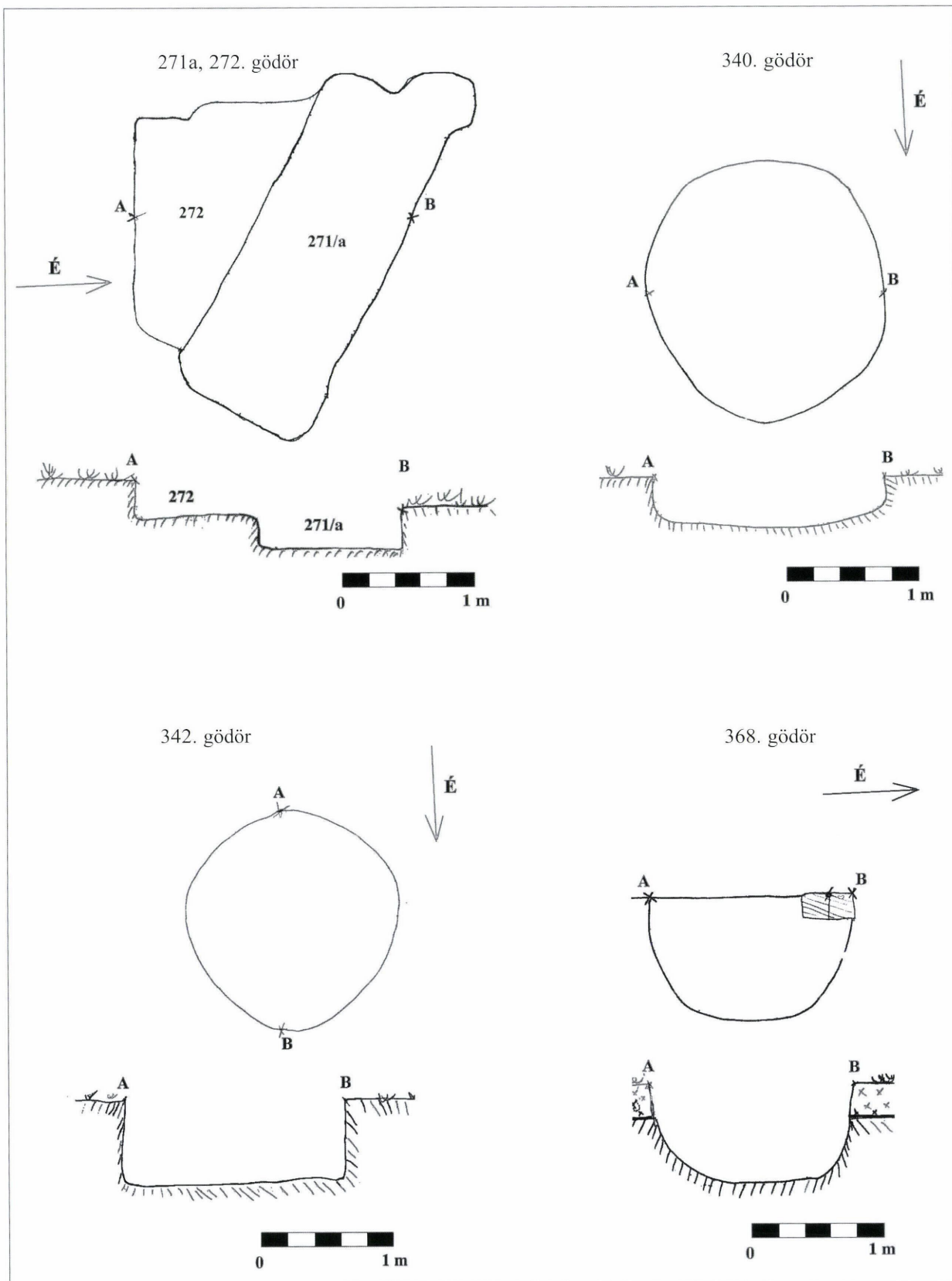
12. kép Szegvár-Kontra-part – a 271a, 272, 340, 342 és 368. gödrök alap és metszetrajza Fig. 12. Szegvár-Kontra-part, ground plan and section of the pits Nr. 271a, Nr. 272, Nr. 340, Nr. 342, Nr. 368.
