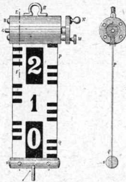
4. sz. rajz. Cséti-féle vagy selmeczi szintező szalag.
