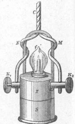
2. sz. rajz. Cséti-féle elektromos függő lámpa.
