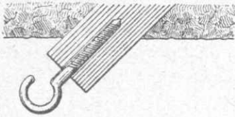
1. sz. rajz. Cséti függélyező csavarja.
