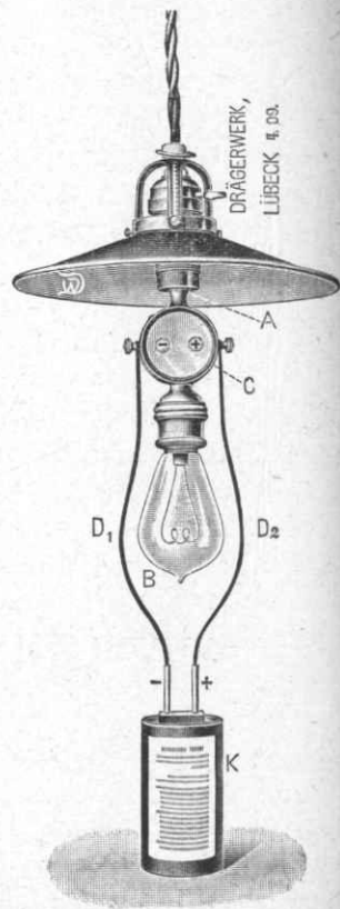
2. sz. rajz. A Dräger-féle vilámlamos biztonsági sisaklámpa töltőszerkezete.
