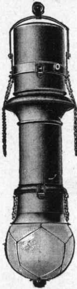
2. sz. rajz. Láng ivlámpa lefelé irányított, ferde elrendezésű hátszénpálcákkal.
