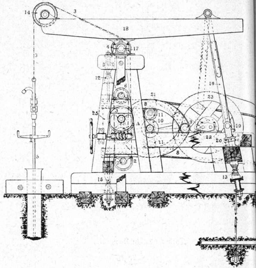
A »Rationell« rendszerű géberendezés.
