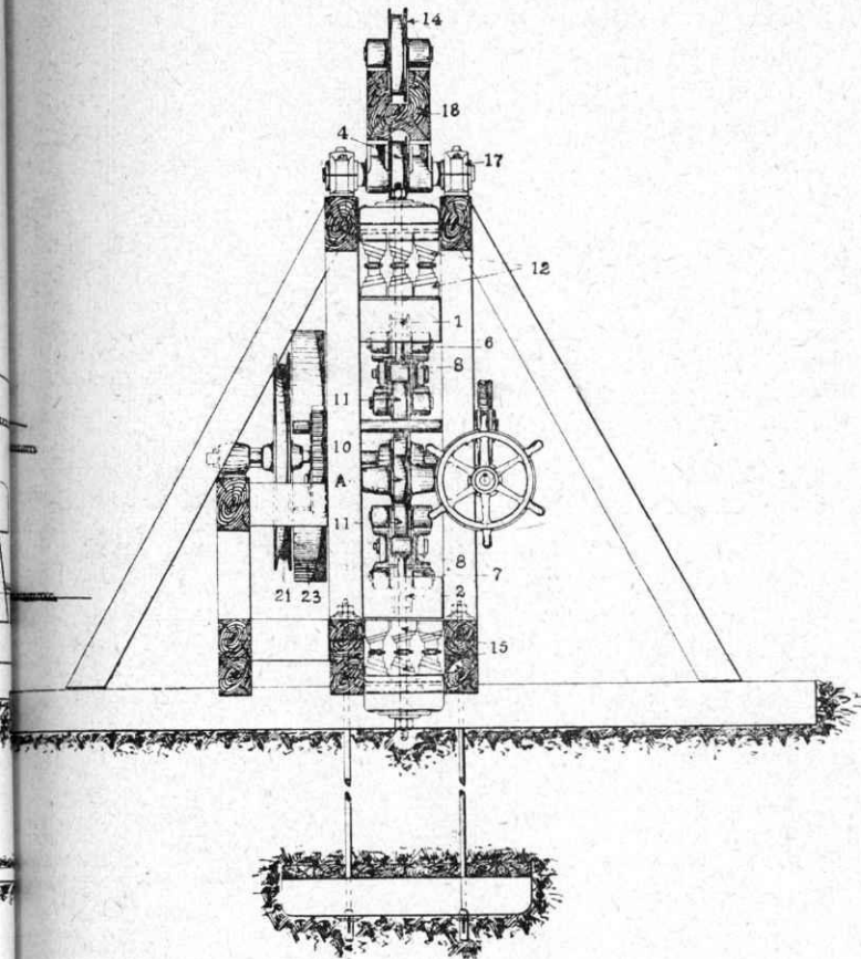
A »Rationell« rendszerű géberendezés.
