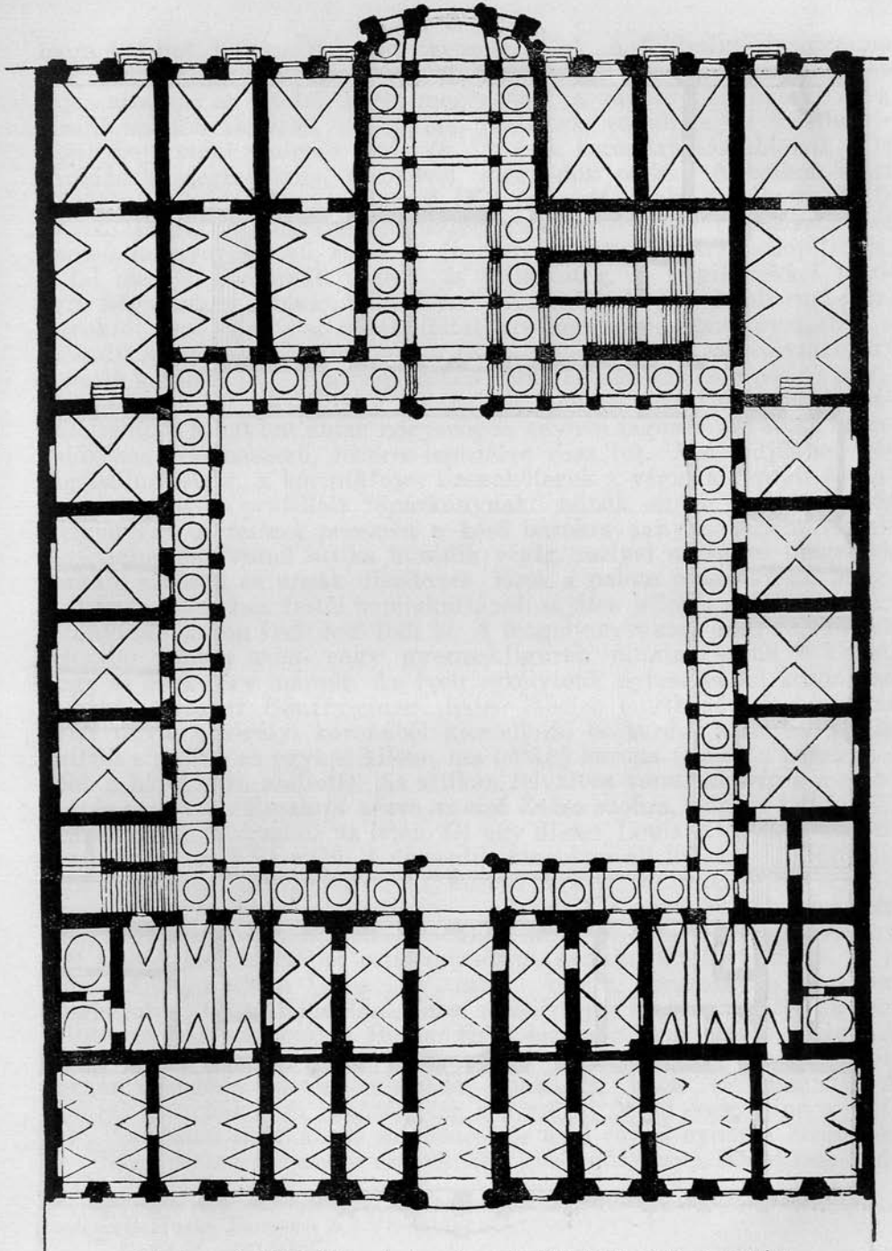
A kolozsvári Bánffy-palota rekonstruált földszinti alaprajza. (Lépték: cca 1:400. Felmérte és rajzolta a szerző.)
