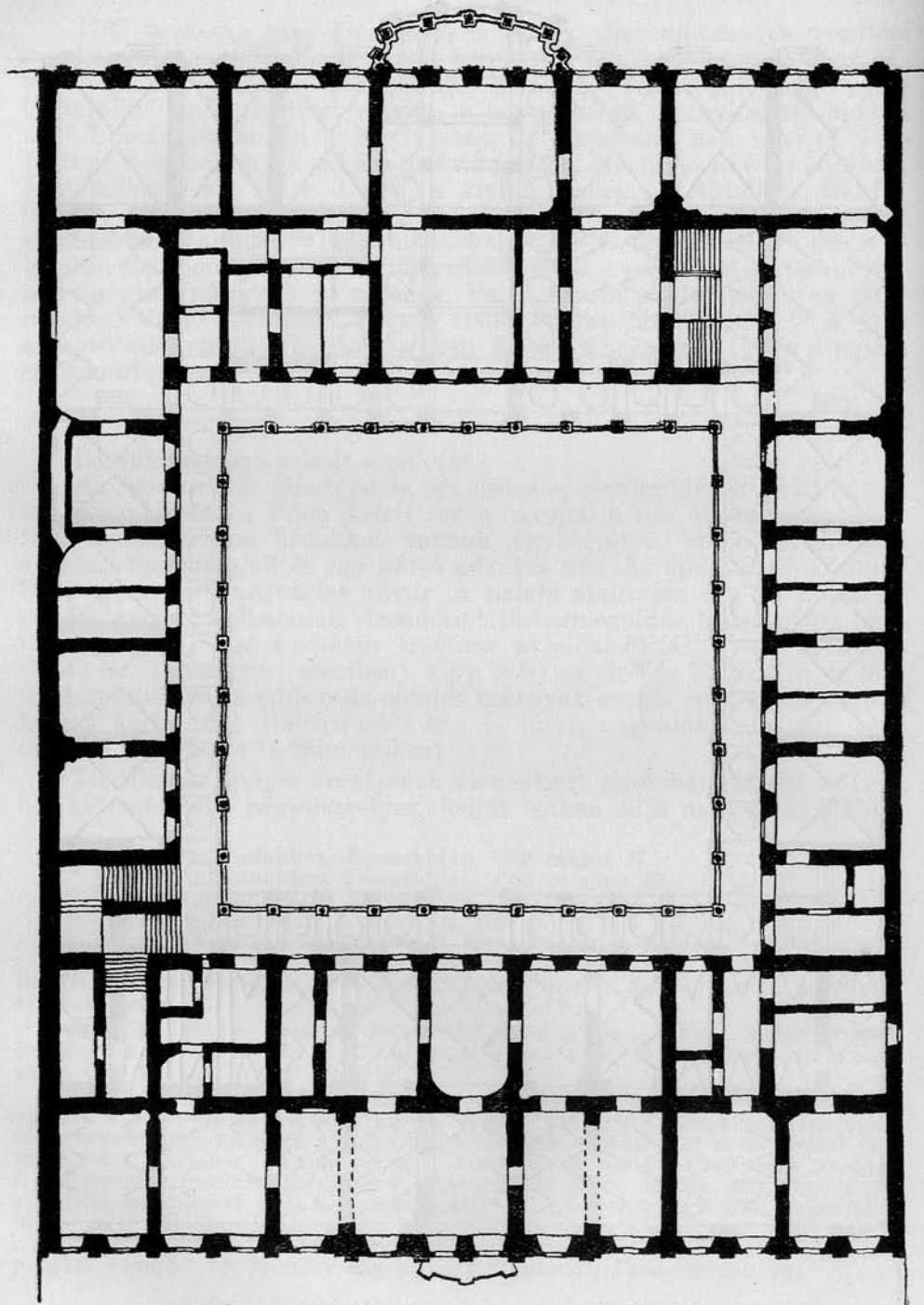
A kolozsvári Bánffy-palota emeleti alaprajza. (Lépték: cca 1:400. Felmérte és rajzolta a szerző.)
